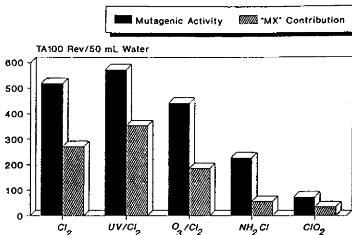
Figure 1 Activité mutagène (Rev./50 mL) et contribution du MX à la mutagénicité calculée dans l'eau du lac Savojärvi (COD: 20 mg/L) après traitement avec divers désinfectants.
