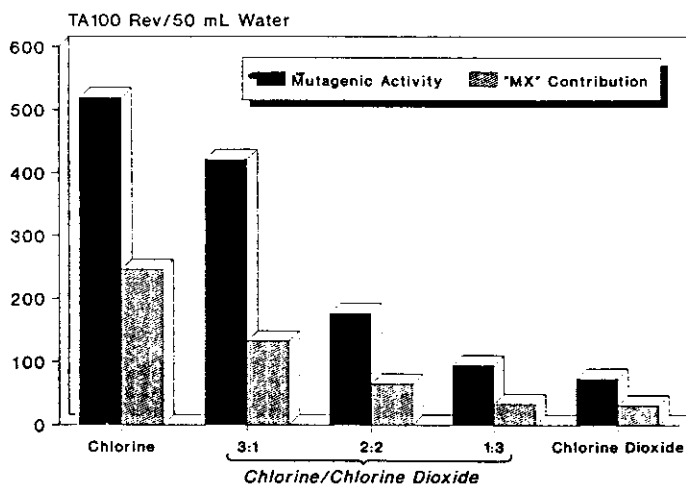
Figure 4 Activité mutagène (Rev./50 mL) et contribution du MX à la mutagénéité calculée dans l'eau du lac Savojärvi après traitement à différentes valeurs de chlore/dioxyde de chlore. Concentration initiale de désinfectant : 20 mg/l.
