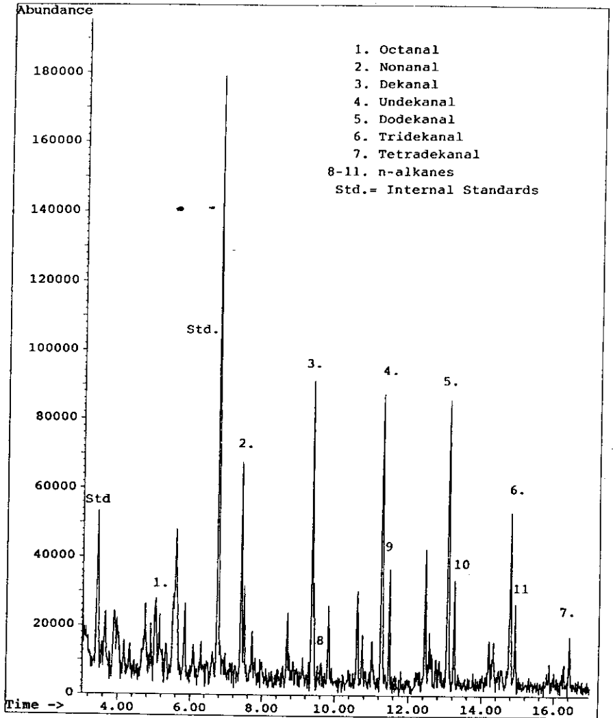
Figure 7 Chromatogramme des sous-produits organiques volatils formés lors d'une désinfection UV de l'au du lac Savojärvi Temps d'irradiation : 6 heures.
