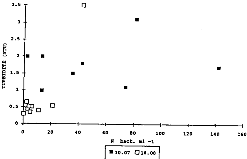
Figure 5 Turbidité en fonction du nombre de bactéries. Turbidity versus bacteria quantity.
