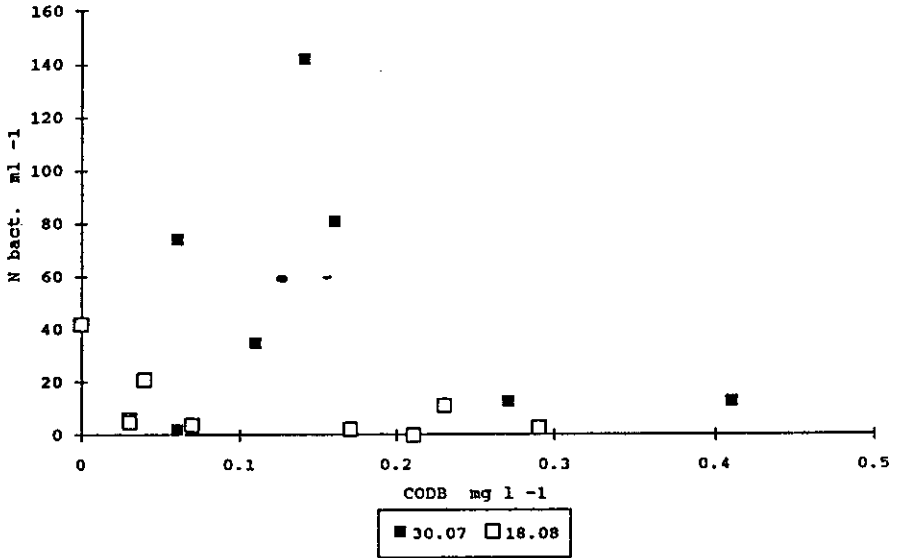
Figure 6 Nombre de bactéries en fonction du CODB. Bacteria quantity versus CODB.
