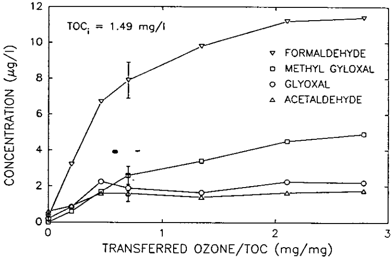
Figure 1 The impact of ozone dose on the formation of aldehydes. Effets de l'ozone sur la formation des aldéhydes.
