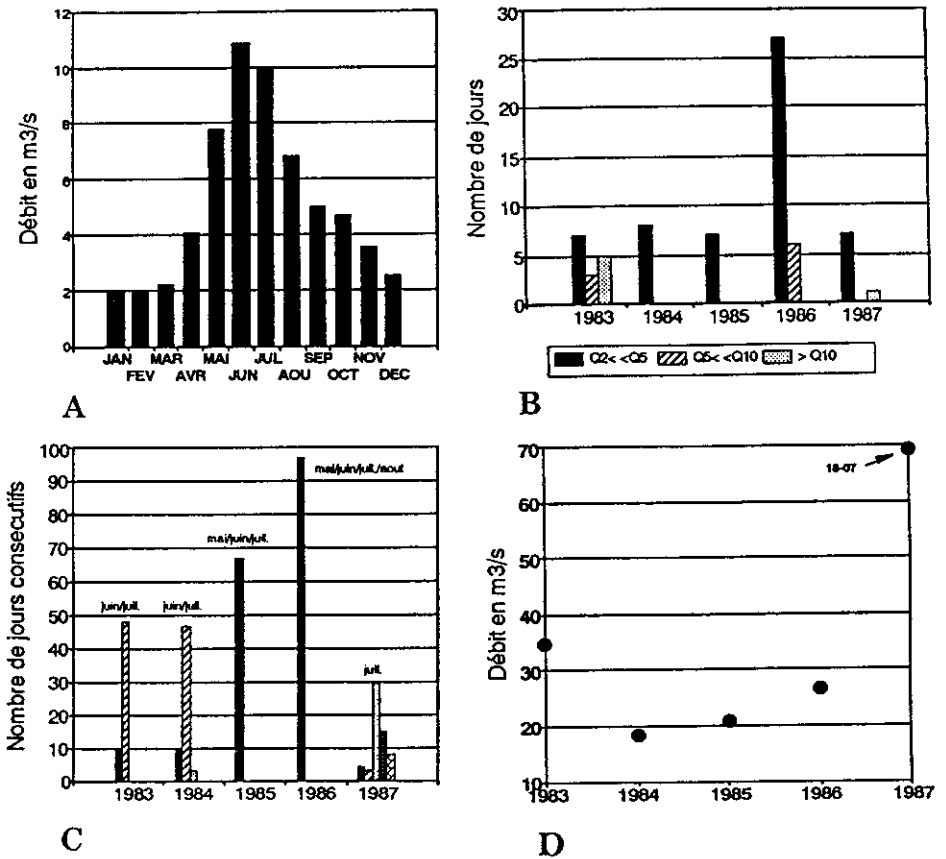
Figure 5 Exemples de données hydrologiques utilisées dans le cadre d'une étude globale de la capacité d'accueil physique d'un cours d'eau. Ici la Séveraisse à Villar Loubière (05).
