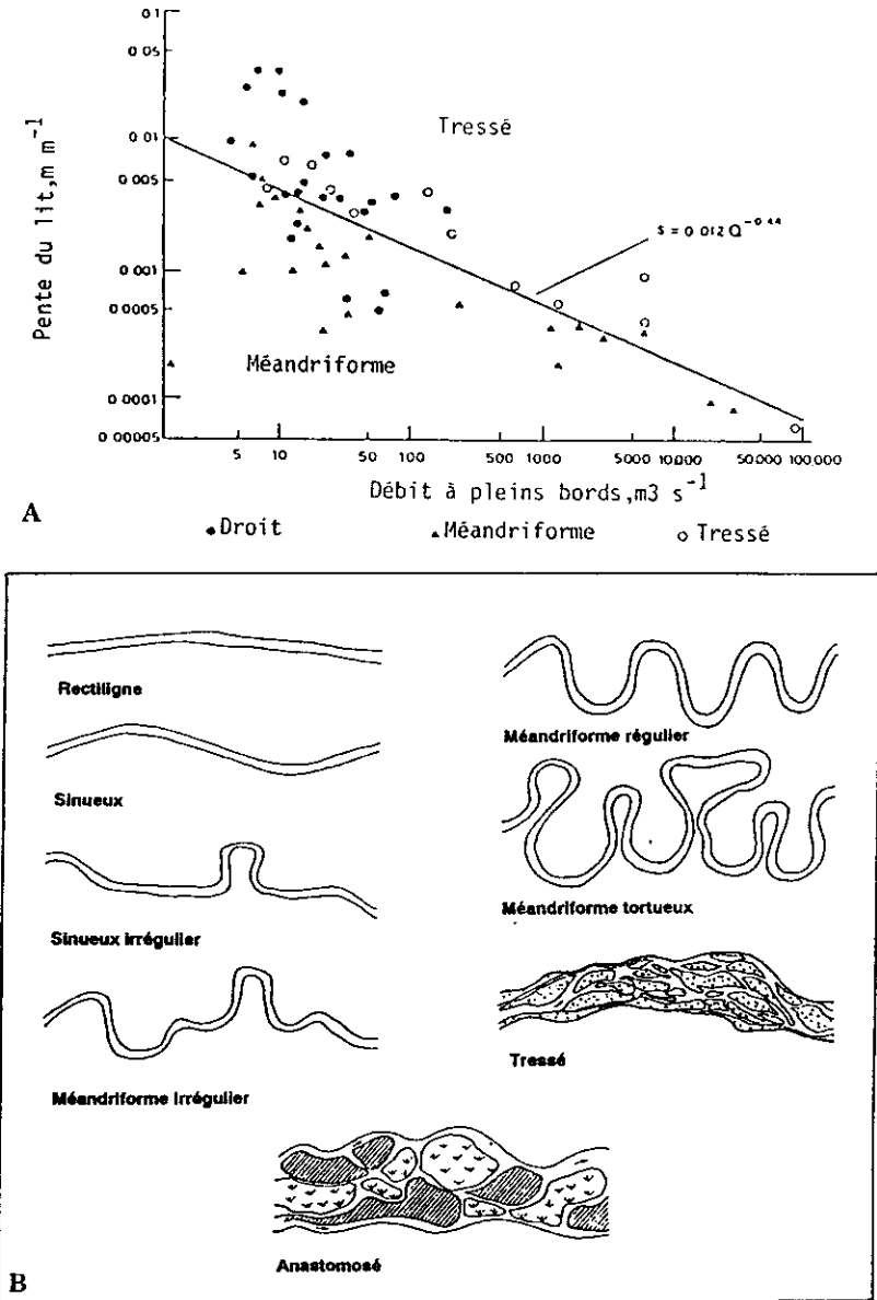
Figure 1 A. Distinction entre modèles tressé et méandriforme sur la base d'un rapport pente/débit (d'après LÉOPOLD & WOLMAN, 1957). B. Les différents types de modèles fluviaux. A. Distinction between braiding and meandering on the basis of slope/discharge ratio. B. Channel patterns.
