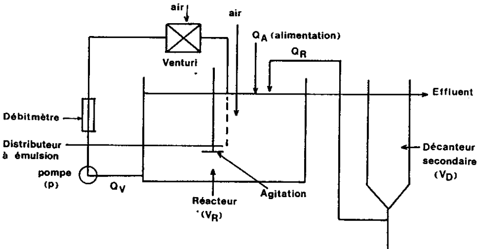
Figure 1 Représentation schématique du pilote.
