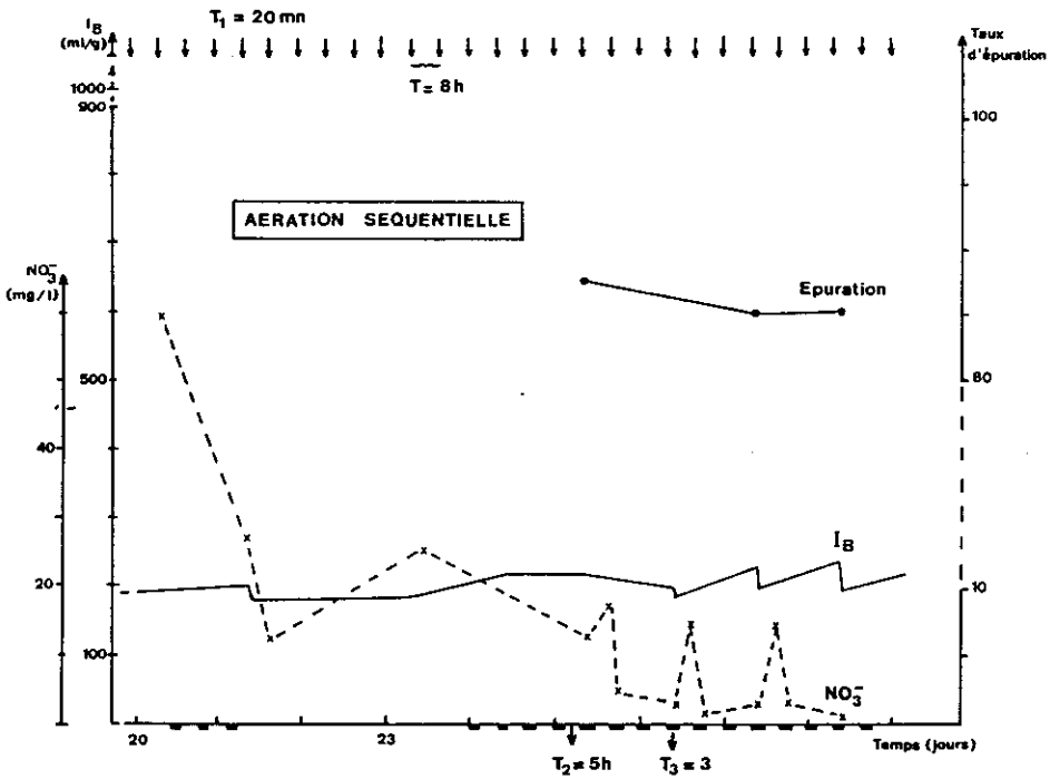
Figure 6 Evolution de l' I_B , DCO et \text{NO}_3^- en fonction du temps pour Re = 0,71 \cdot 10^5 , T_1 = 20 mn, T = 8 h (aération séquentielle).
