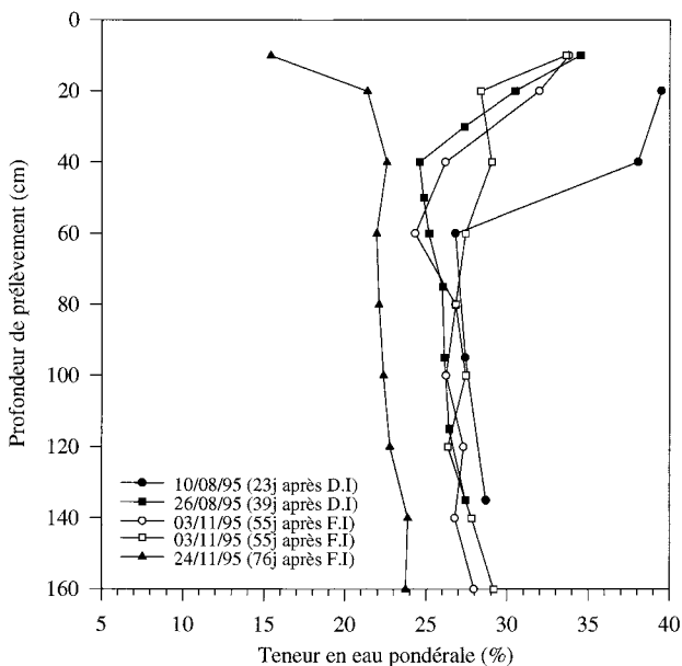
Figure 7 Évolution de la teneur en eau pondérale à P4 (D.I et F.I : début et fin d'irrigation). Humidity profiles at P4 (D.I and F.I: beginning and end of irrigation).
