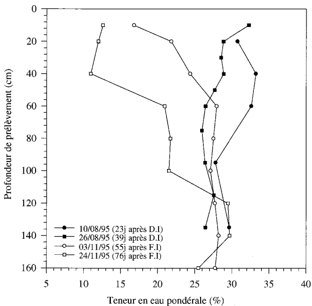
Figure 8 Évolution de la teneur en eau pondérale à P2 (D.I et F.I : début et fin d'irrigation). Humidity profiles at P2 (D.I and F.I: beginning and end of irrigation).
