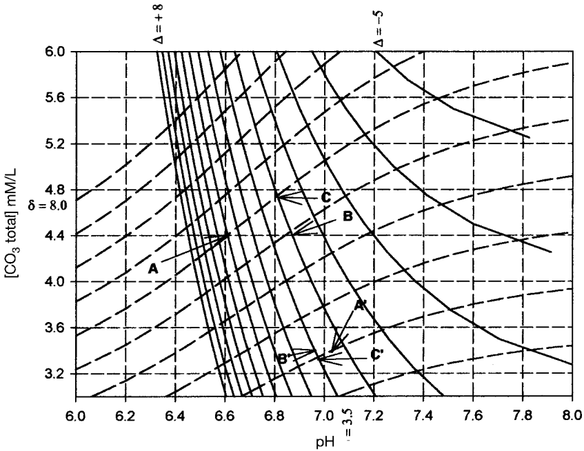
Figure 6 Élimination de CO 2 par aération. CO 2 removal by aeration.
