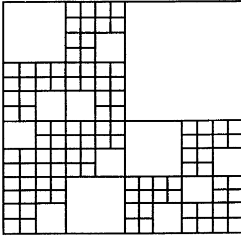
Figure 2 Modèle fractal de fragmentation de dimension 1,59 (in TURCOTTE, 1992). (les lignes de différentes longueurs simulent les fractures de différentes tailles) Fractal model of fragmentation with dimension of 1.59 (in TURCOTTE, 1992). (lines of different lengths represent the fractures of different sizes)
