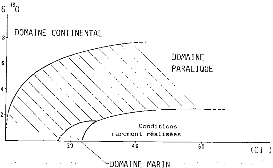
Figure 15.- Essai de délimitation des eaux marines, paraliqes et continentales, dans le contexte géographique et climatique égyptien à partir de leurs teneurs en oxygène-18 et en \text{Cl}^- .
