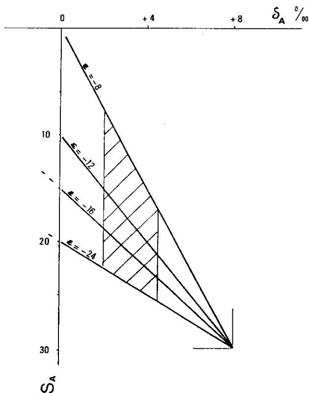
Figure 12.- Valeurs de \delta_A et de S_A en fonction de \epsilon . Zone hâchée : zone des valeurs vraisemblables.
